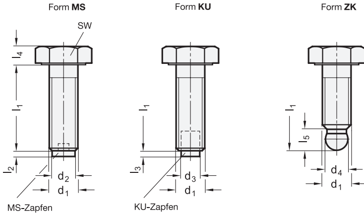
Druckstück GN 631 / GN 631.5
