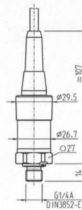
mit Kabelausgang IP 67
