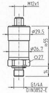
mit Rundstecker M12 x 1 (4-polig)
