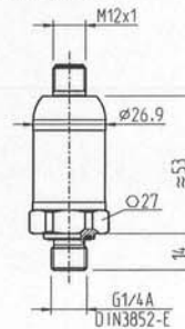
mit Rundstecker M12 x 1 (4-polig, metallisch)
