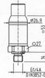
mit Kabelausgang 1/2 NPT Conduit
