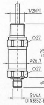
mit Kabelausgang 1/2 NPT Conduit
