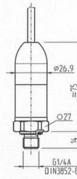
mit Kabelausgang IP 68, FEP, IP 6K9K
