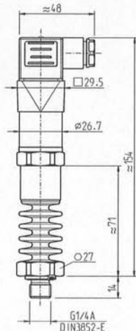
mit Winkelstecker DIN 175301-803 A und Kühlstrecke
